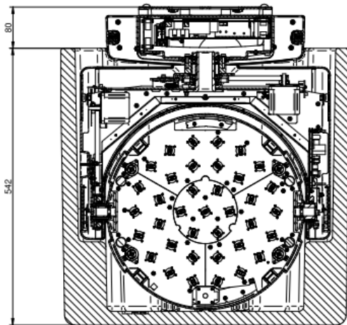
SEZIONE A-A
